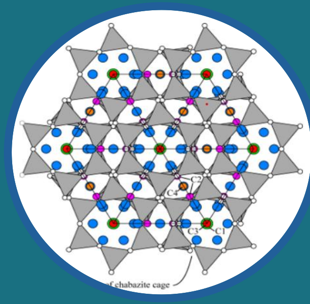
Chabazite
