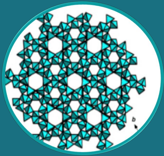
Analcime
